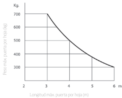
Para accionadores con vástago de 400 mm
