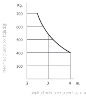
Para accionadores con vástago de 265 mm
